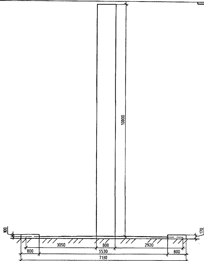
Вид спереди
