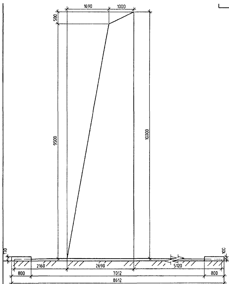
Вид сбоку
